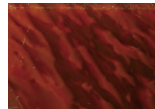
▲ 自然銅のサイズが小さければアベンチュリン効果を現さず、銅のコロイドによって赤色を形成します
