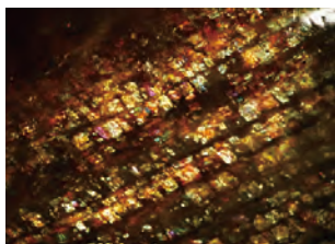
▲ オリゴクレス・サンストーンに見られる鱗辺状の赤鉄鉱の内包物
